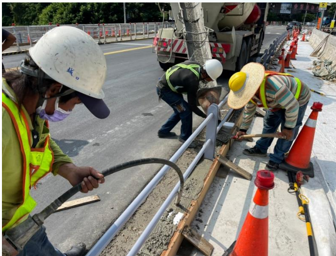
防護欄杆與基礎施作
