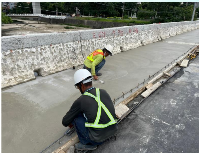
噴花地坪結構混凝土澆置
