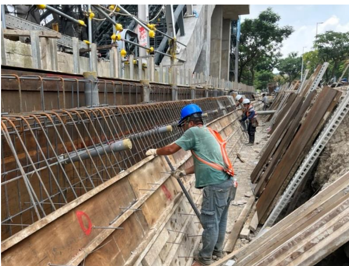
第二升層模板組立
