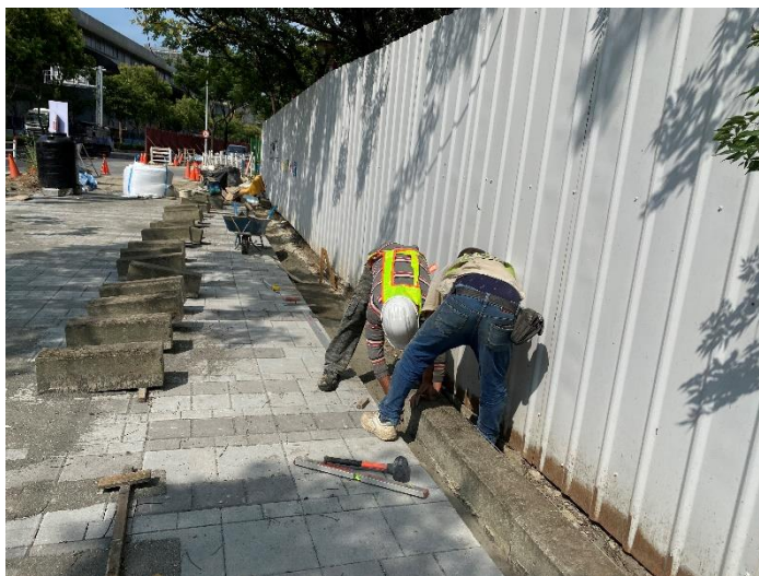
既有樹圍石調整
