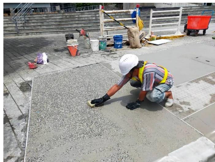
陶博館前斜坡道施作
