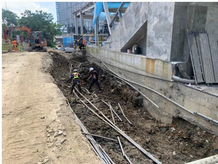
新設擋土牆開挖與管障清除
