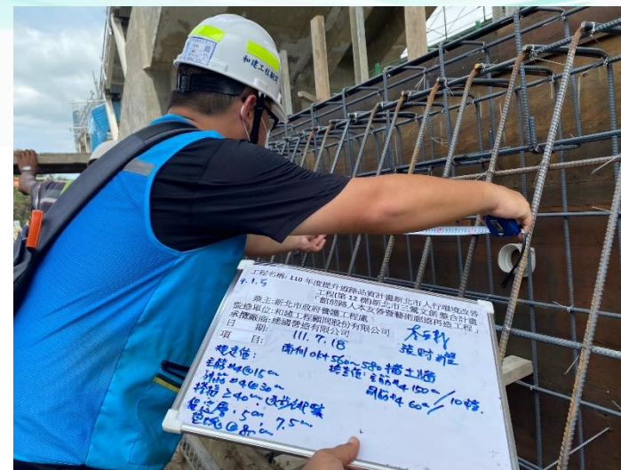
鋼筋組立與施工抽查
