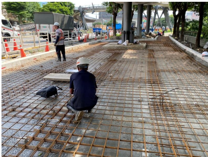
人行道結構層施作
