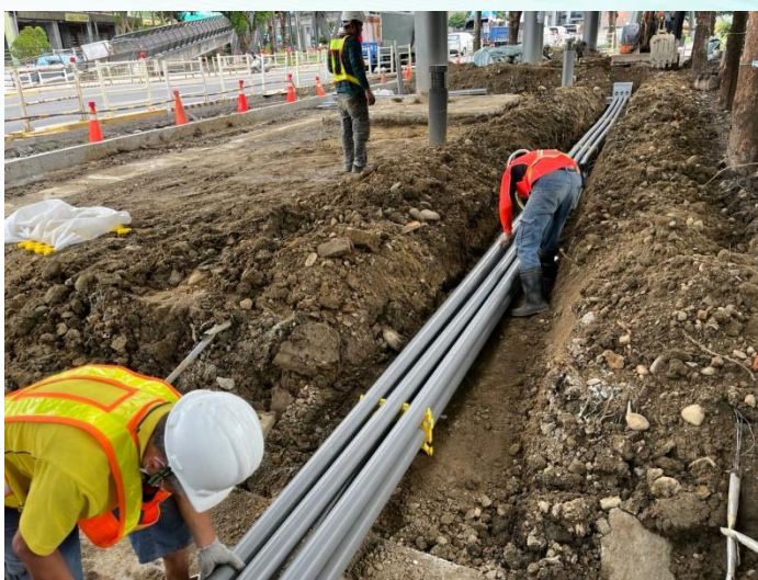
弱電管溝管材組立
