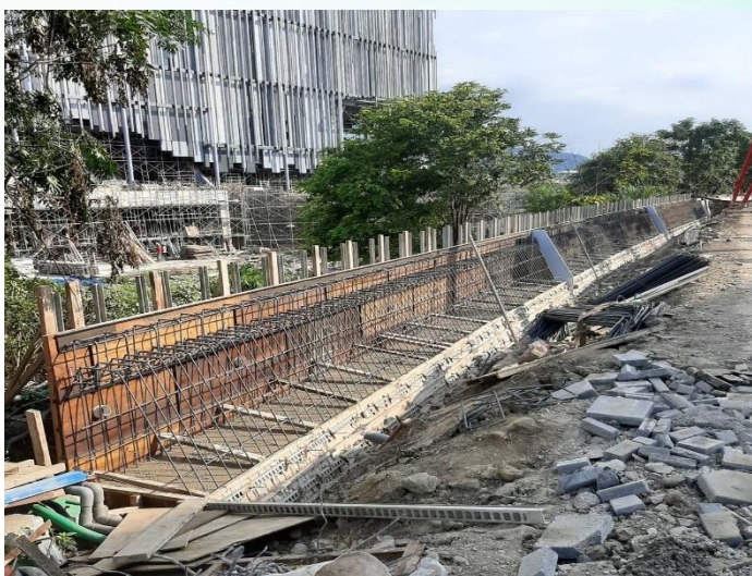
新設擋土牆基礎開挖
