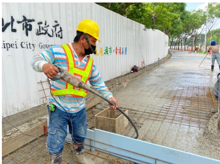
人行道結構層混凝土澆置
