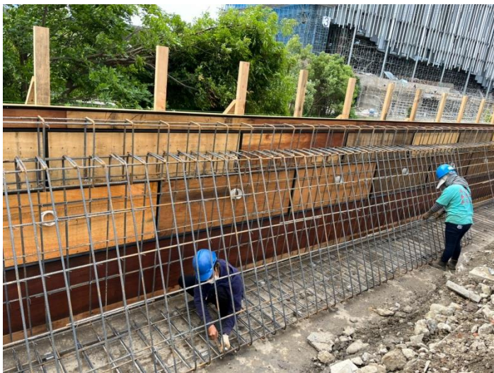
新設擋土牆鋼筋綁紮組立
