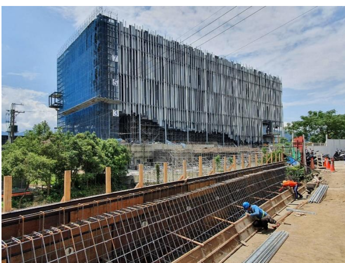
新設擋土牆內模組立
