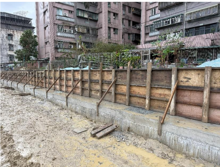
U2新設擋牆施作
