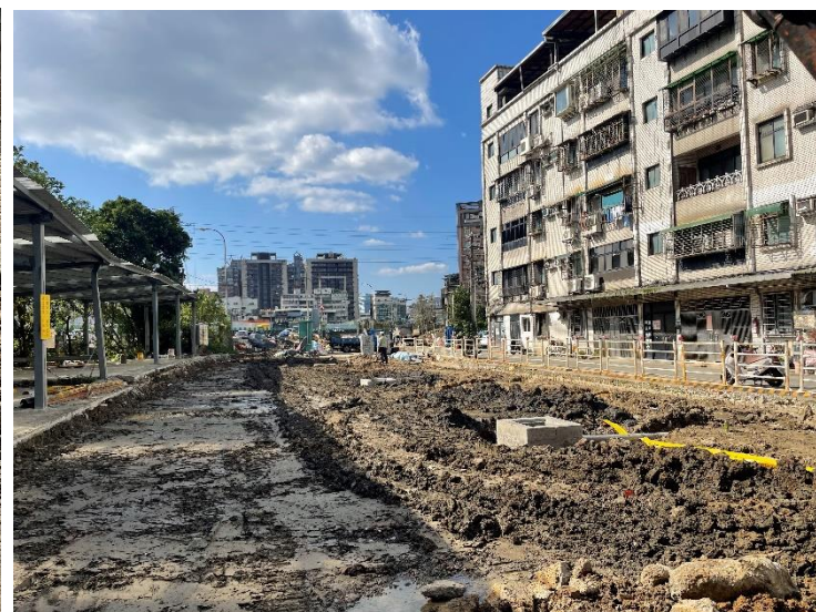
湖前街二巷鋪面整理及集水井預埋
