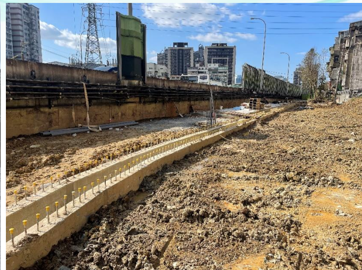
U4段新設側溝完成後現況
