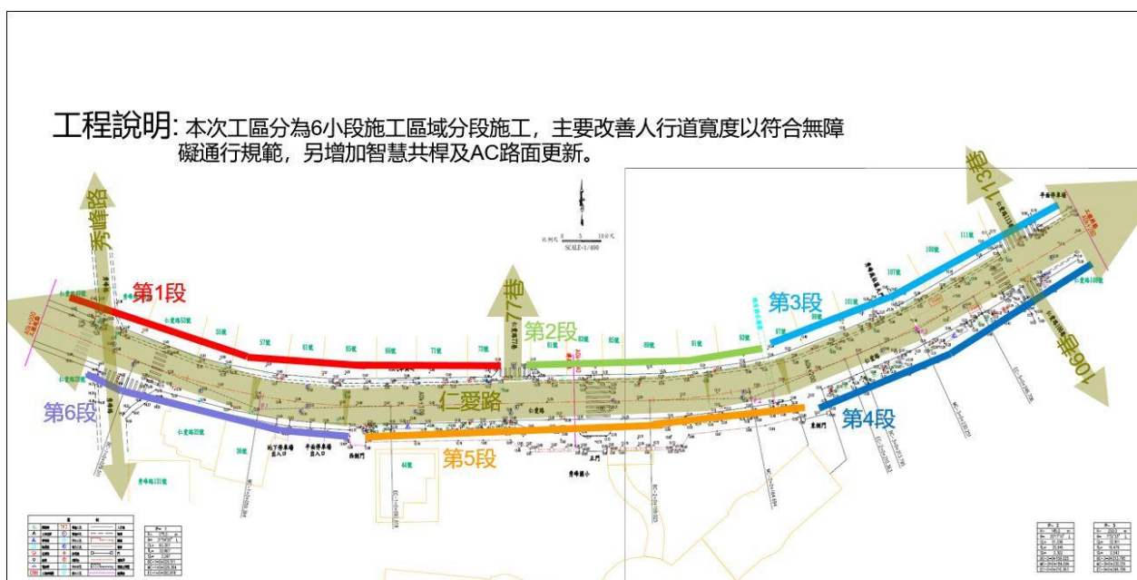
(6) 平面圖
