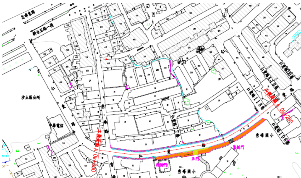
(6) 平面圖
